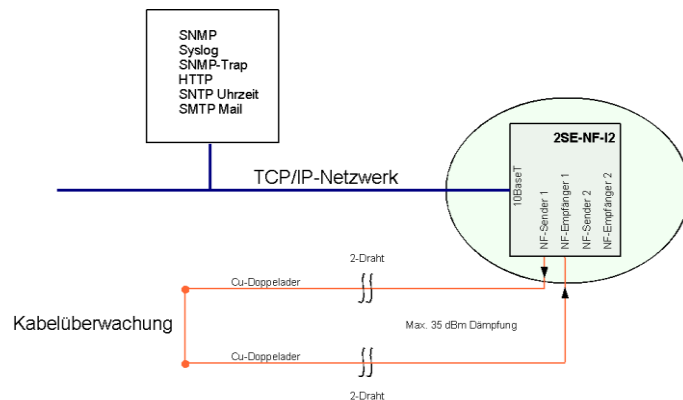
Abbildung 1: Kabelüberwachung
