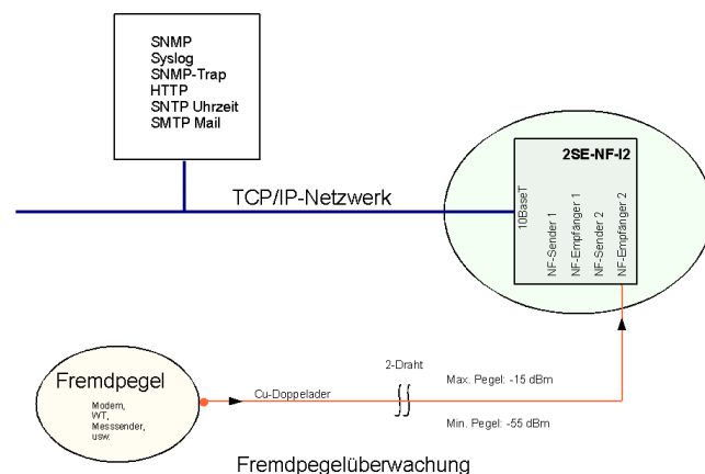
Abbildung 2: Fremdpegelüberwachung
